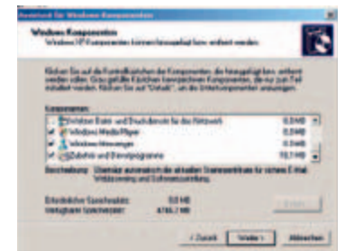
Abb. 6 Windows-Komponenten
